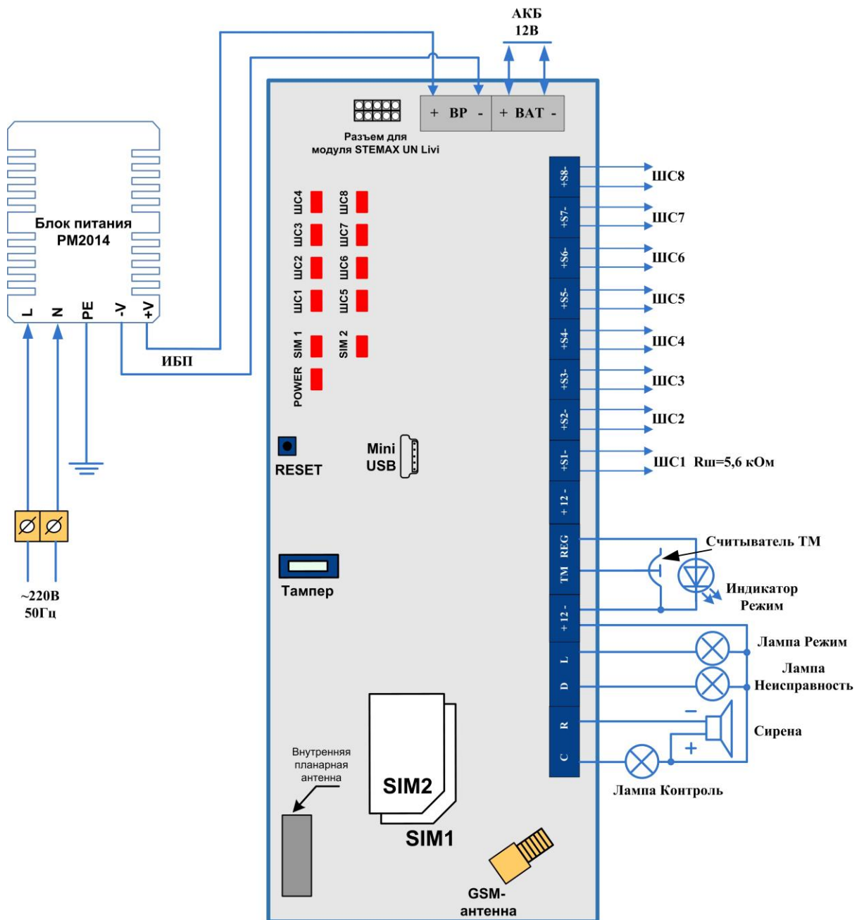
Рисунок А.2 —Схема внешних подключений контроллера
