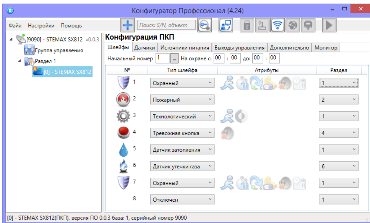
Рисунок 4.33 — Вкладка Шлейфы
