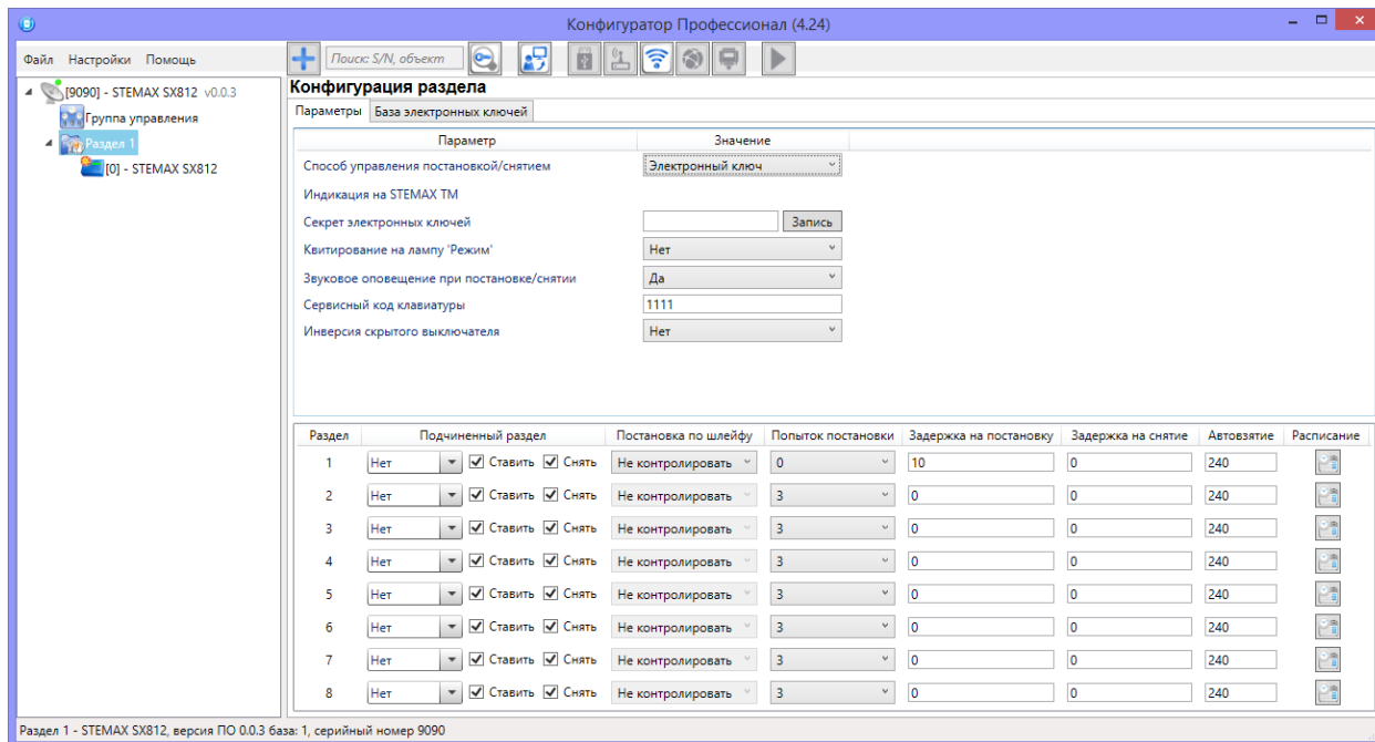
Рисунок 4.26 — Вкладка Параметры
