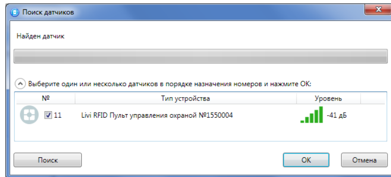
Рисунок 4.37 — Поиск радиоустройства
